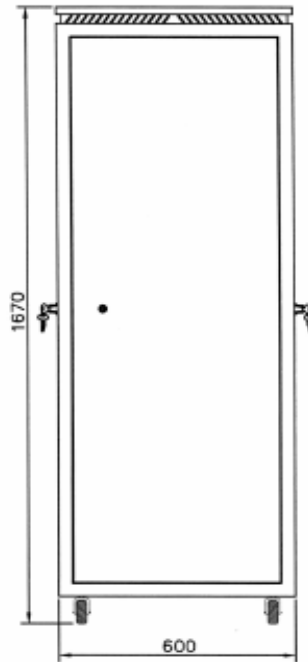
ARKA GÖRÜNÜS
