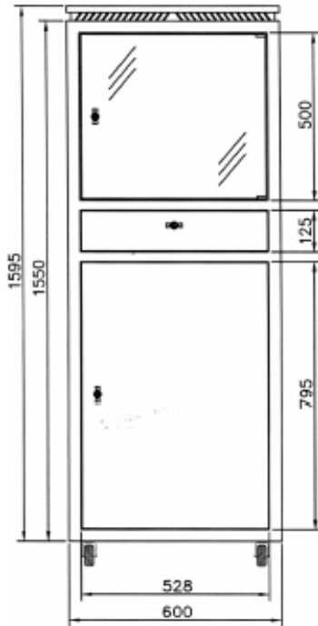
ÖN GÖRÜNÜS
